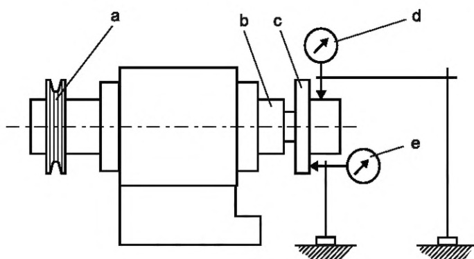
a — ременный шкив; b — шпиндель; c — оправка; d — измерительная головка 1; e — измерительная головка 2
