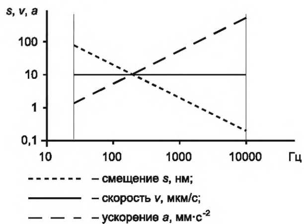
Рисунок В.1 — Соотношение амплитуд на различных частотах при амплитуде виброскорости 10 мкм/с
