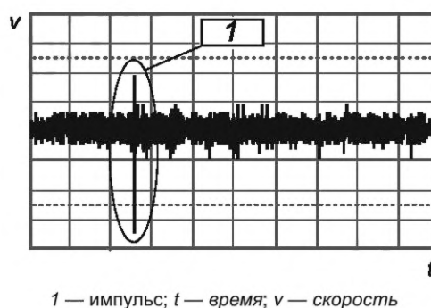
Рисунок 1 — Пример импульса во временной области
