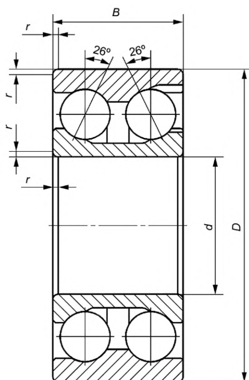
Рисунок 1 — Конструктивное исполнение 05
