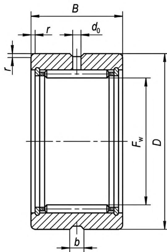
Рисунок 6 — Конструктивное исполнение 35
