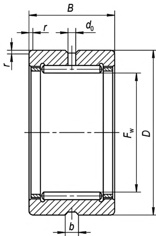
Рисунок 4 — Конструктивное исполнение 25
