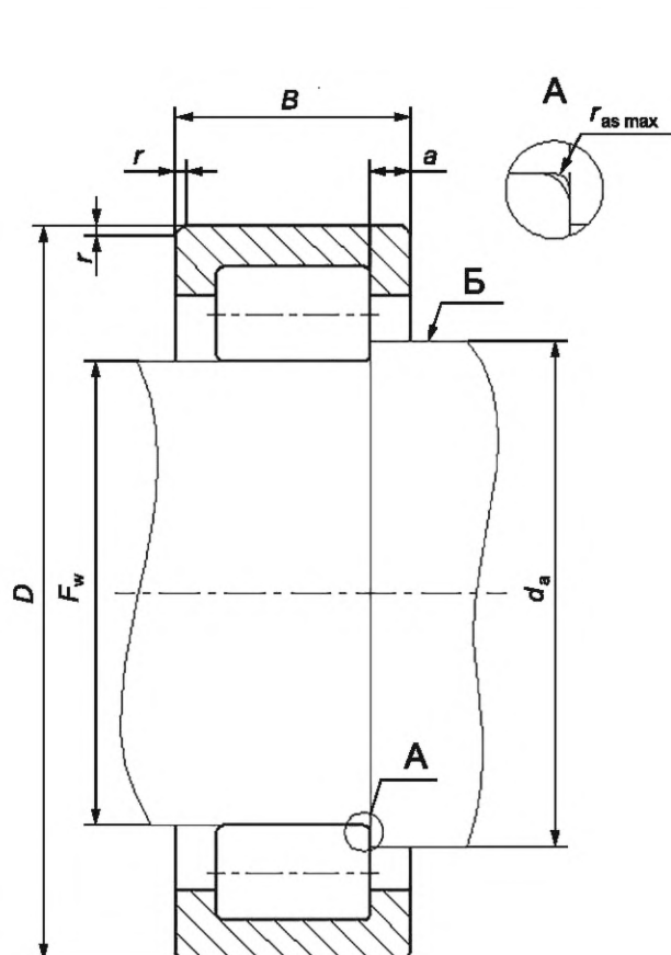
Рисунок 1 — Конструктивное исполнение 29
