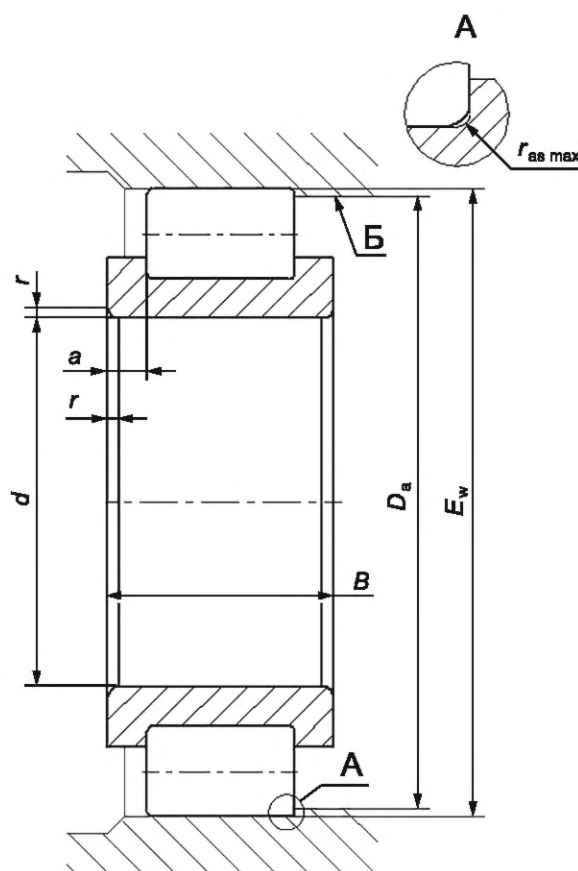
Рисунок 2 — Конструктивное исполнение 50
