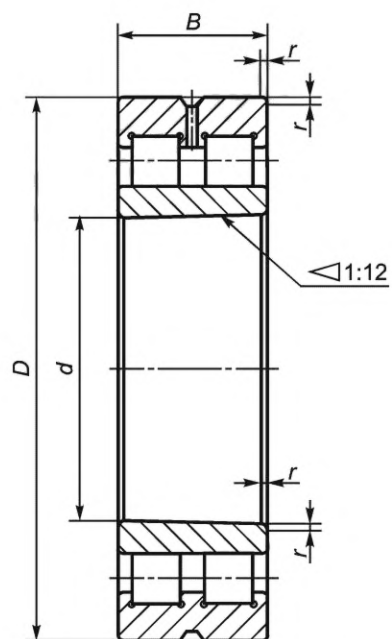
Рисунок 2 — Конструктивное исполнение 16K
