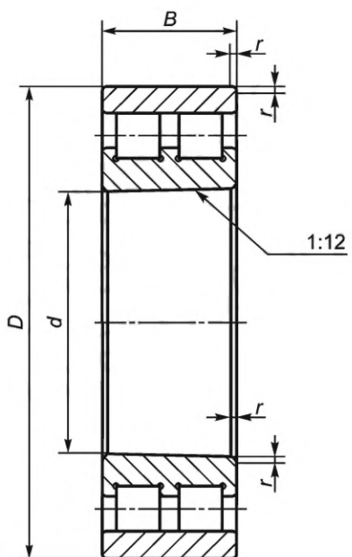
Рисунок 3 — Конструктивное исполнение 18
