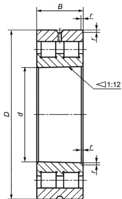
Рисунок 4 — Конструктивное исполнение 18K
