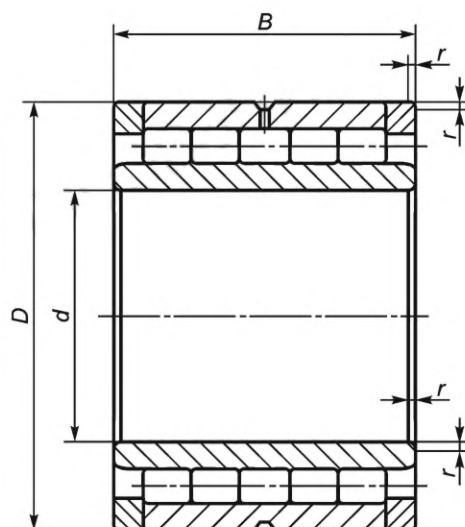
Рисунок 10 — Конструктивное исполнение 45К
