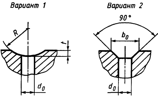
d 0 — диаметр отверстия для смазки; R — радиус кольцевой канавки; t — глубина канавки; b 0 — ширина канавки
