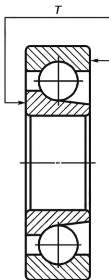
Рисунок 6 — Обозначение монтажной высоты
