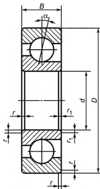
Рисунок 2 — Конструктивное исполнение 07
