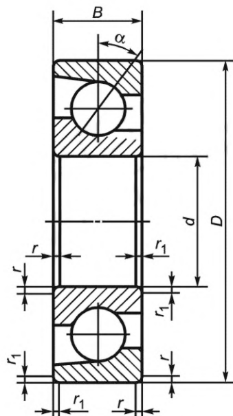
Рисунок 5 — Конструктивное исполнение 02
