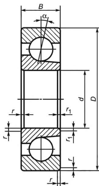
Рисунок 4 — Конструктивные исполнения 03K7, 03K, 04K, 06K
