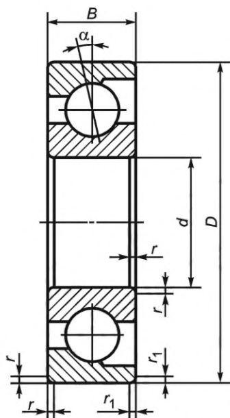
Рисунок 1 — Конструктивное исполнение 00
