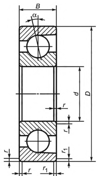
Рисунок 3 — Конструктивные исполнения 03, 03K6, 04, 06
