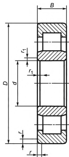
Рисунок 3 — Конструктивное исполнение 03
