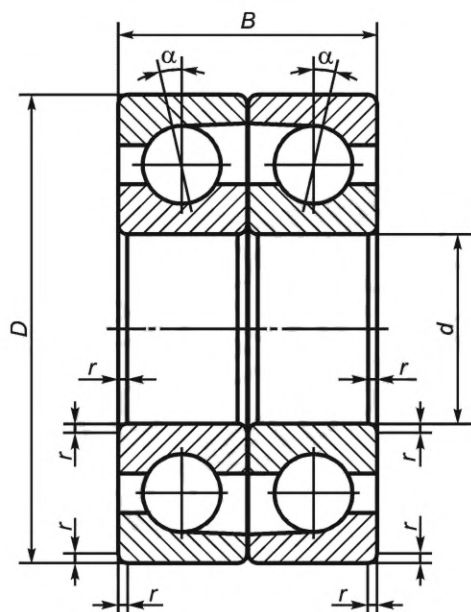
Рисунок 5 — Конструктивные исполнения 33, 34, 36
