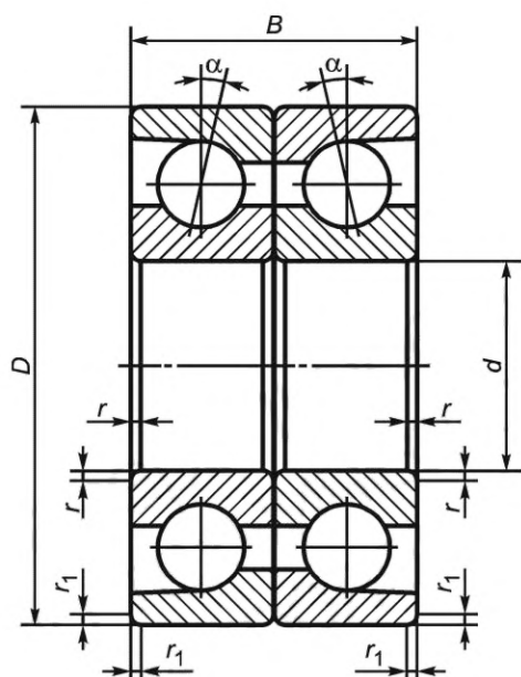
Рисунок 3 — Конструктивные исполнения 23, 24, 26
