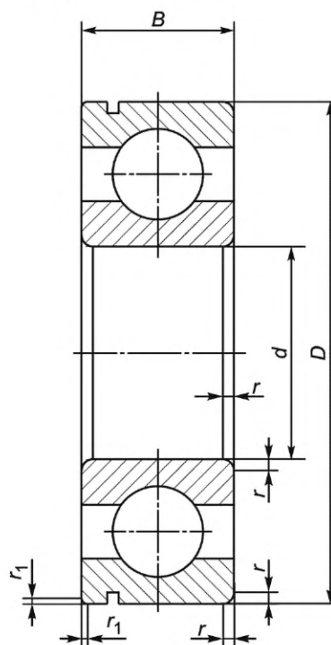
Рисунок 2 — Конструктивное исполнение 05
