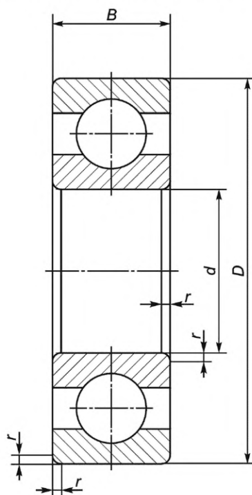
Рисунок 1 — Конструктивное исполнение 00
