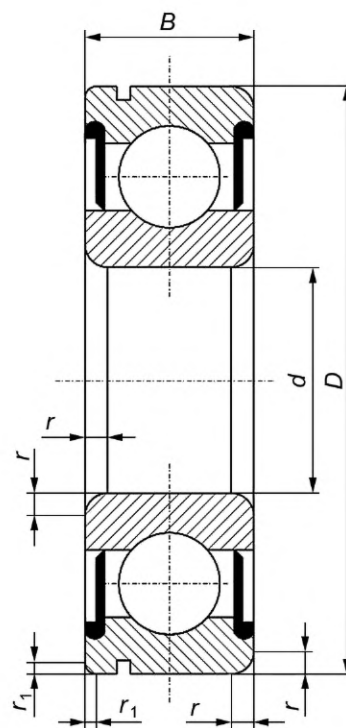
Рисунок 4 — Конструктивное исполнение 75
