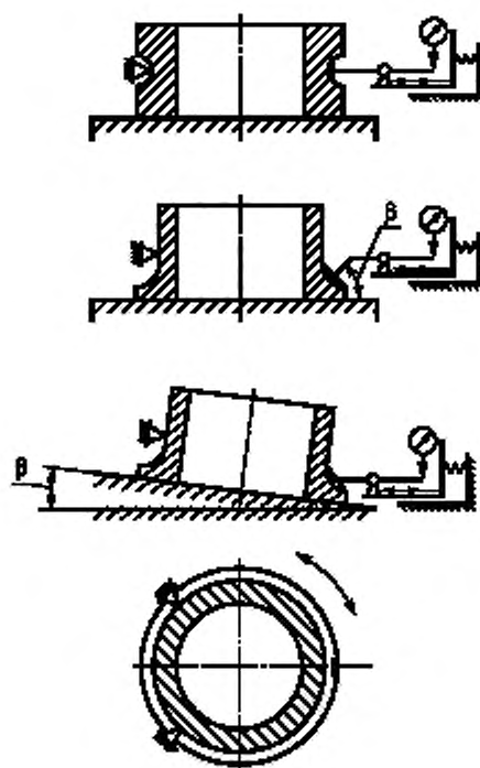
β — угол наклона наконечника или опорной плоскости (конструктивно)
