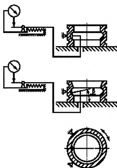
\beta — угол наклона измерительного наконечника (конструктивно)
