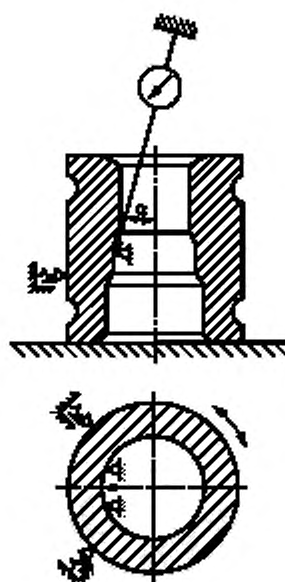
\alpha — угол наклона оси измерительной головки относительно оси кольца
